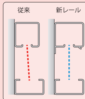
新レール断面
