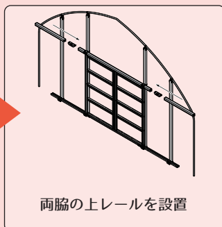
中央の上レールを設置した後、滑車を取り付けたドアを横から入れる。
